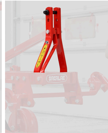
Traktör Orta Kol Bağlantısı Tractor Middle Arm Connection
